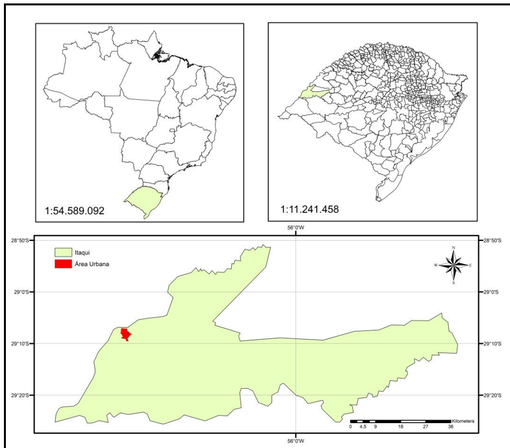
Figura 1 - Localização da área estudada.
