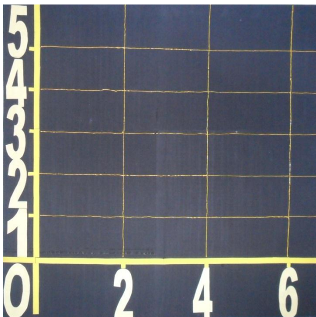
FIGURA 36 - Gráfico da velocidade em função do tempo ( v \times t )
