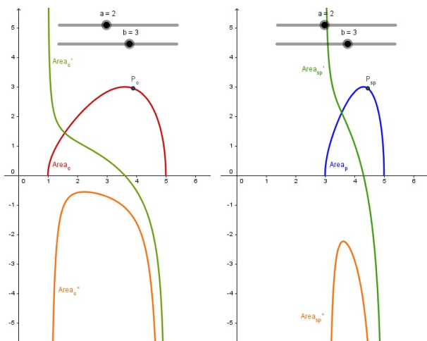
Figura 4.3: Funções área A(p) e A(c) e suas primeira e segunda derivadas
