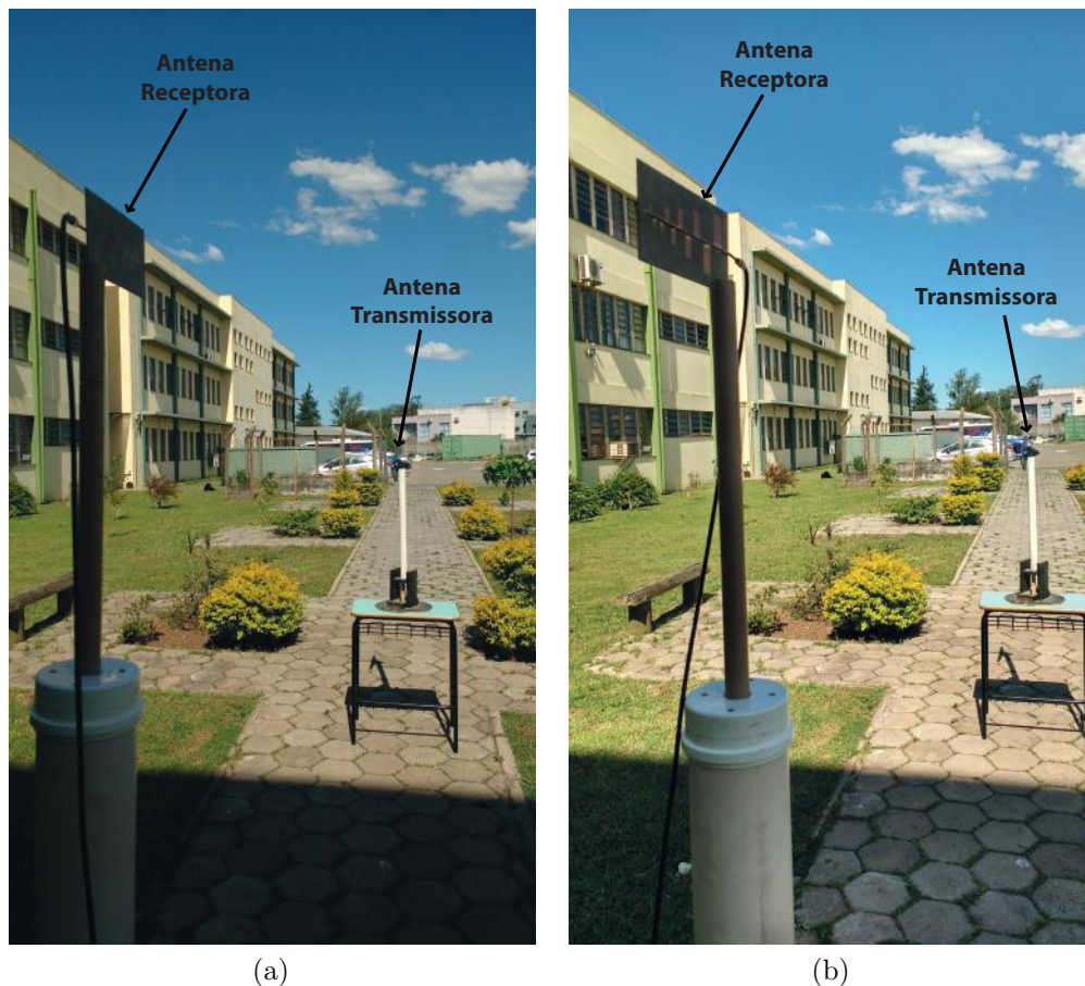
Figura 60 – Medição do plano H (a) antenas em visada direta, (b) rotação da antena receptora de 180^\circ a 360^\circ
