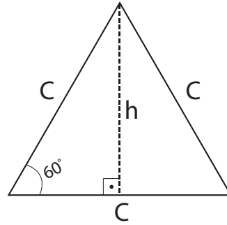
Figura 10 – Triângulo equilátero.
