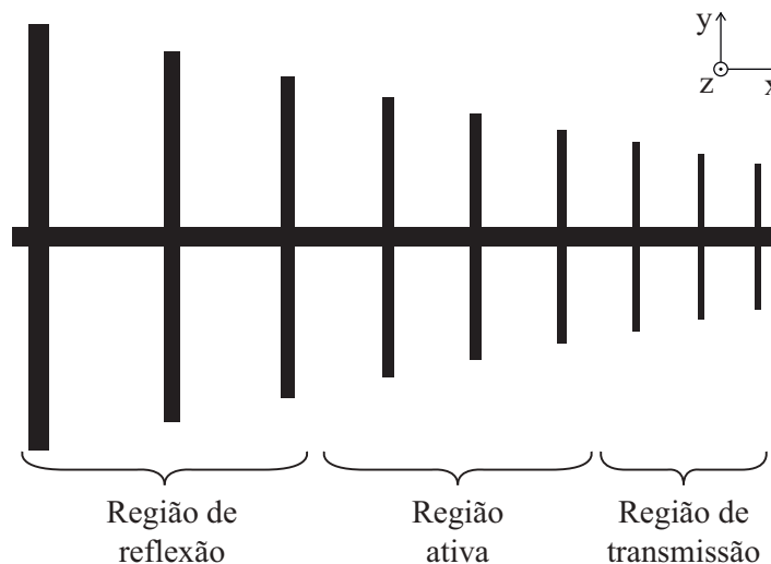
Figura 2 – Regiões de operação da antenna log-periódica.
