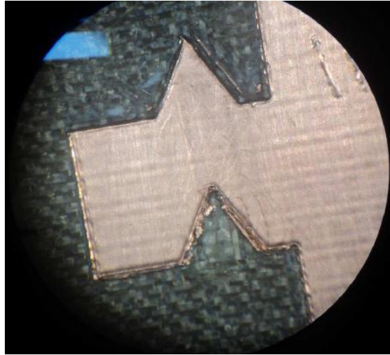
Figura 69 – Dipolo da rede fractal.
